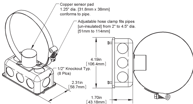
Clamp-On Strap J-Box (JB)
