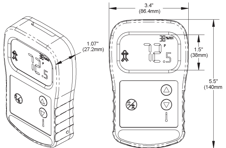
Fig. 1: 3 Button BAPI-Stat
